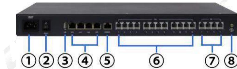
图 1-2 IP PBX800 后面板图
