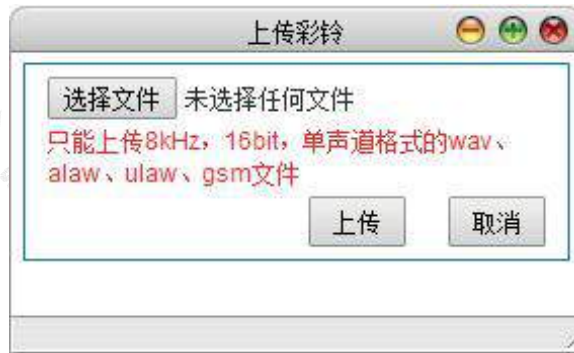
图 6-74 添加提示音
