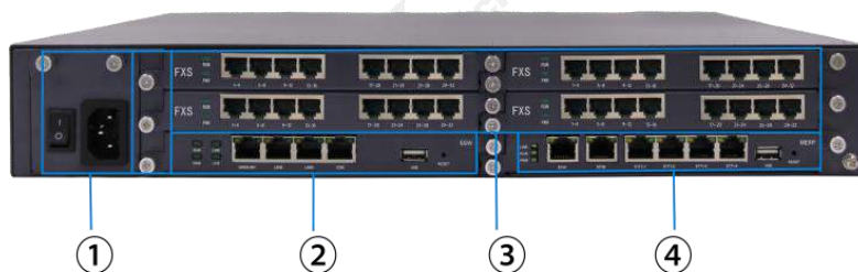
图 1-1 IP PBX3000 前面板图
