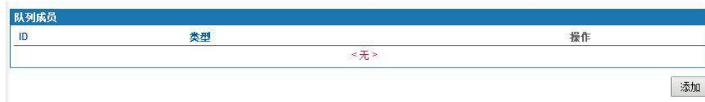
图 6-107 队列成员
