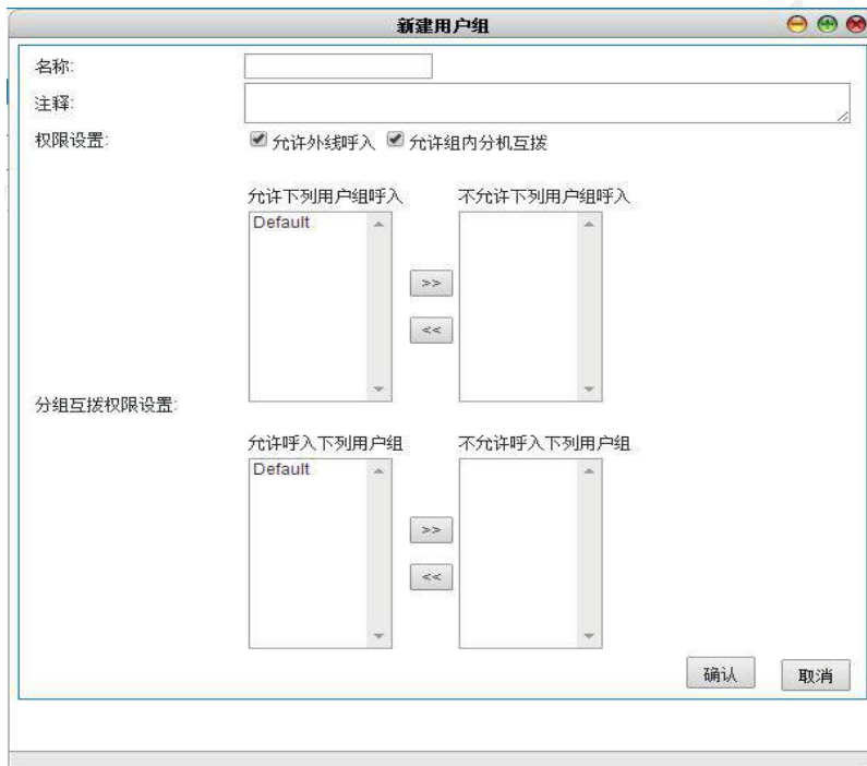
图 6-21 新建用户组
