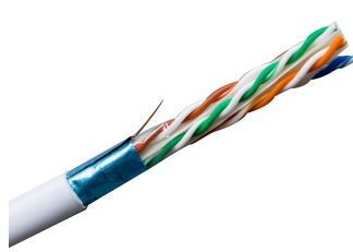
室内超六类铝箔屏蔽网线 Indoor FTP Cat6
