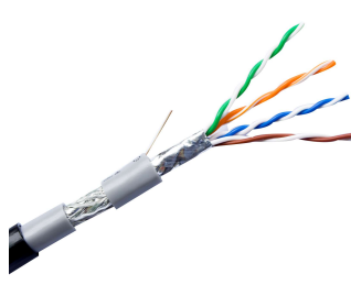
室外超五类铝箔+编织 双屏蔽阻水网线 Outdoor SFTP Cat5e
