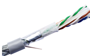
室内超六类铝箔+编织 双屏蔽网线 Indoor SFTP Cat6
