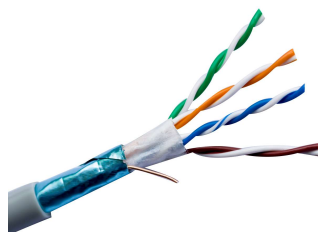
室内超五类铝箔屏蔽网线 Indoor FTP Cat5e
