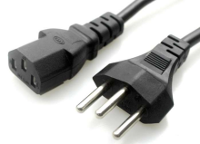
巴西头-品字尾 Brazil-C13
