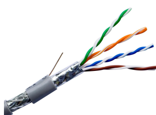
室内超五类铝箔+编织 双屏蔽网线 Indoor SFTP Cat5e
