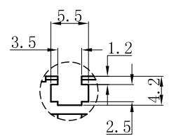
视图A, 比例2:1
