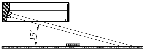
照明示意图
