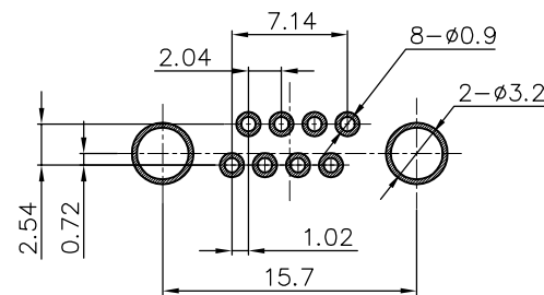
印制线路板示意图 P.C.B. Layout(Top View)
