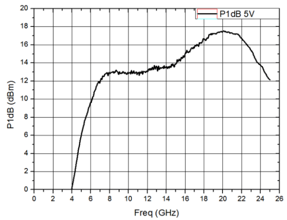
Output P1dB
