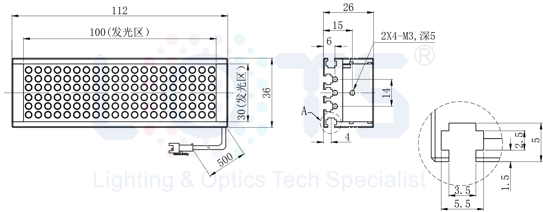
视图A 比例4: 1
