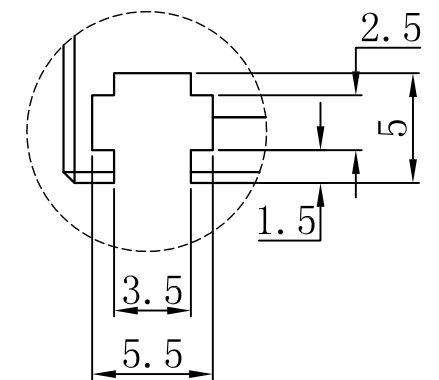
视图A 比例 2:1
