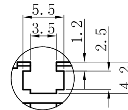
视图A, 比例2:1
