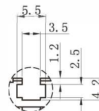
视图A 比例2:1
