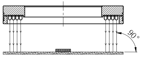
照明示意图
