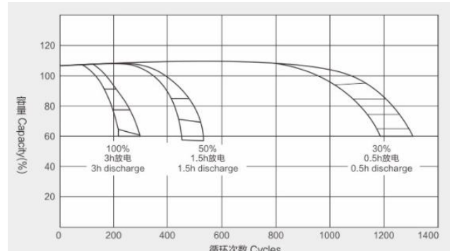
图-6 循环寿命
