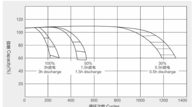
图-6 循环寿命
